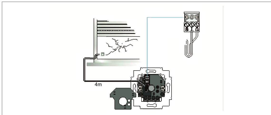
Abb. 2: Angeschlossener Glasbruchmelder
